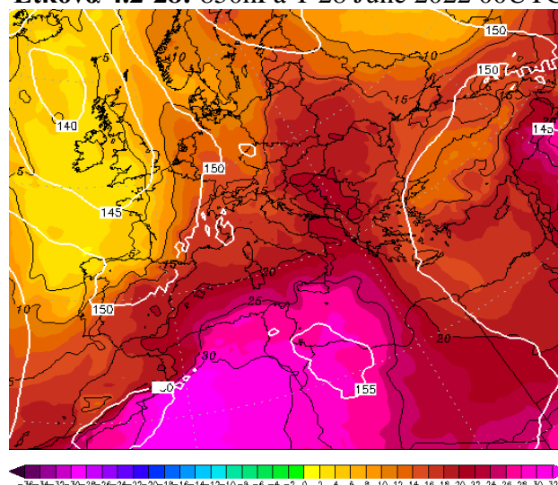
Εικόνα 4.2-30: 850hPa T 30 June 2022 00UTC
