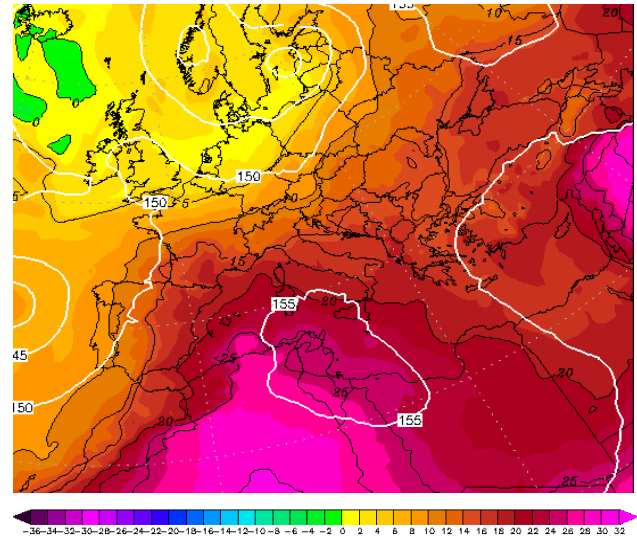
Εικόνα 4.2-2: 850hPa T 2 June 2022 00UTC
