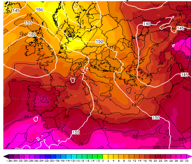
Εικόνα 4.2-40: 850hPa T 10 July 2022 00UTC
