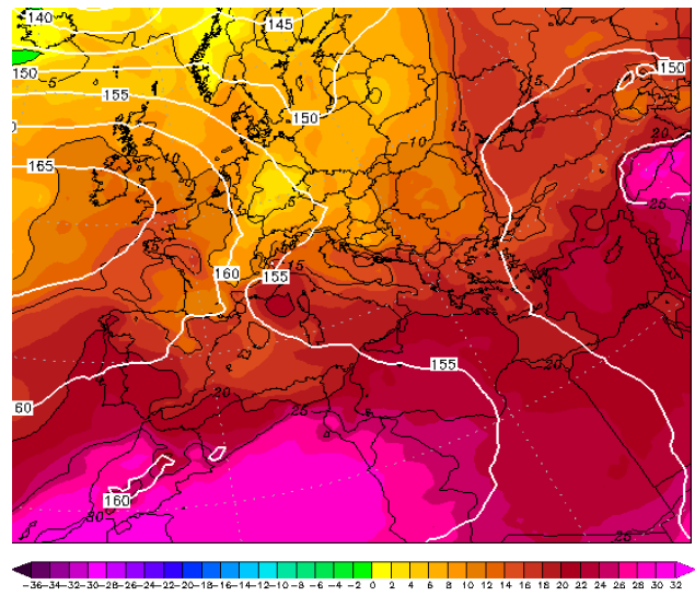
Εικόνα 4.2-38: 850hPa T 8 July 2022 00UTC
