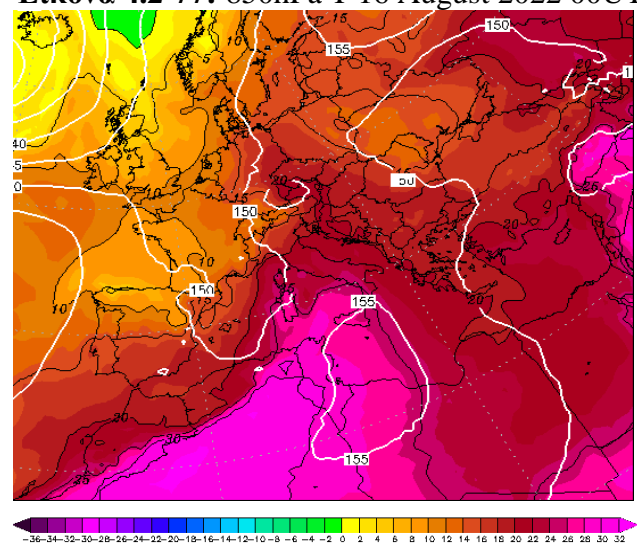
Εικόνα 4.2-79: 850hPa T 18 August 2022 00UTC
