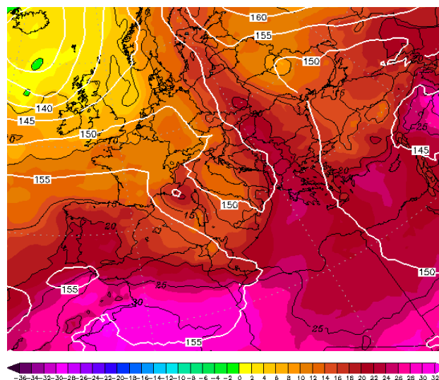
Εικόνα 4.2-81: 850hPa T 20 August 2022 00UTC
