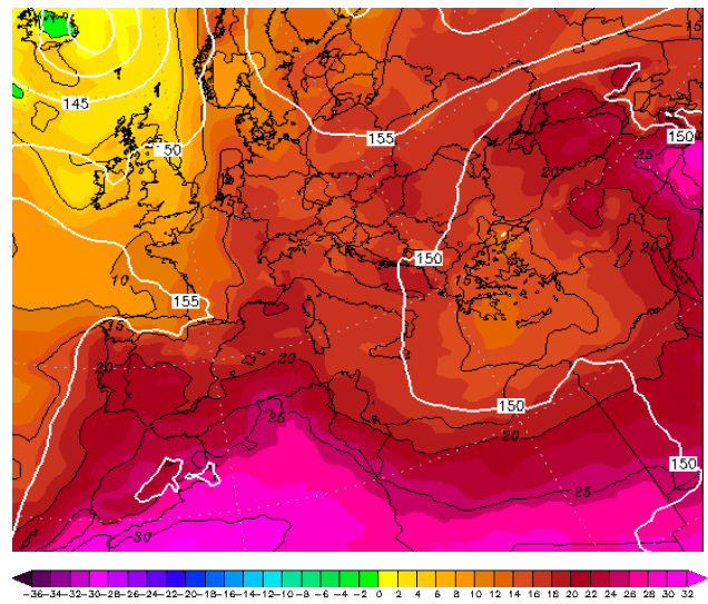
Εικόνα 4.2-87: 850hPa T 26 August 2022 00UTC
