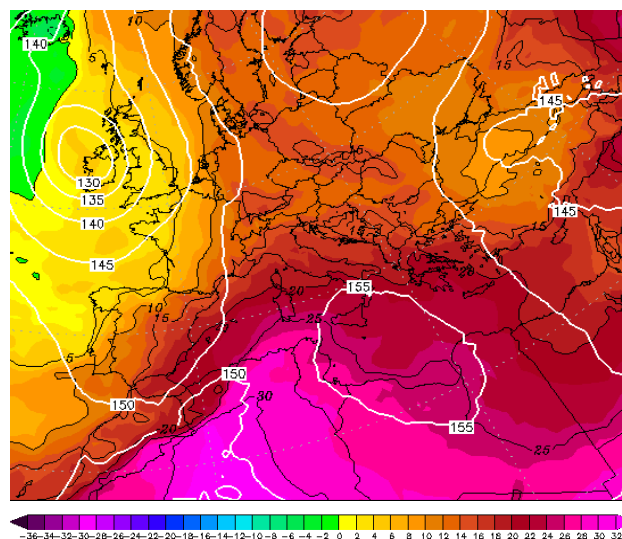
Εικόνα 4.2-26: 850hPa T 26 June 2022 00UTC
