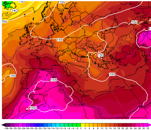
Εικόνα 4.2-74: 850hPa T 13 August 2022 00UTC
