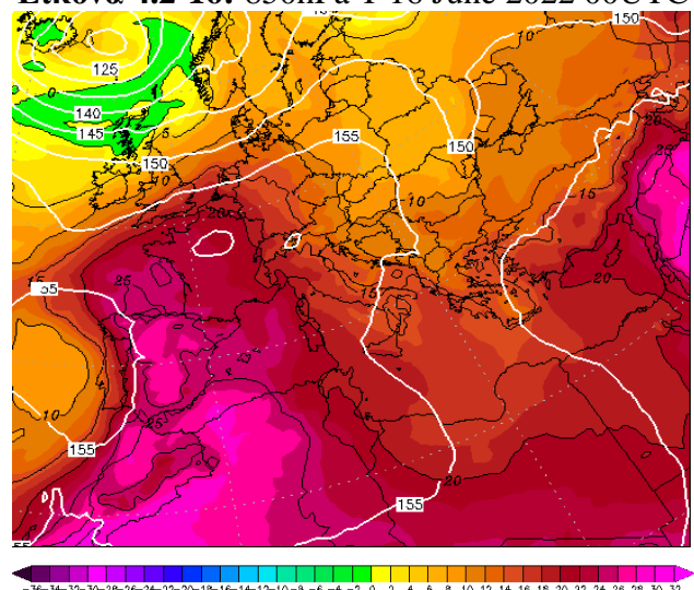
Εικόνα 4.2-18: 850hPa T 18 June 2022 00UTC
