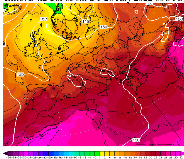
Εικόνα 4.2-58: 850hPa T 28 July 2022 00UTC
