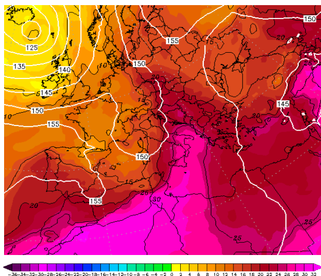
Εικόνα 4.2-80: 850hPa T 19 August 2022 00UTC
