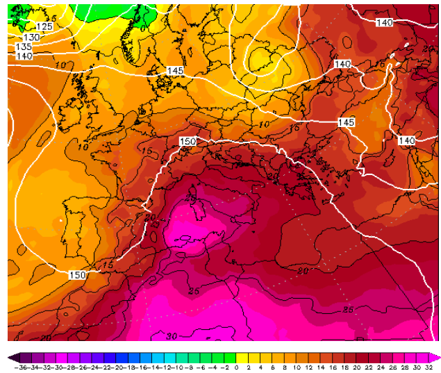
Εικόνα 4.2-22: 850hPa T 22 June 2022 00UTC
