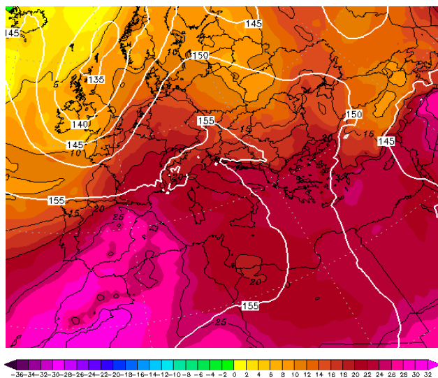
Εικόνα 4.2-55: 850hPa T 25 July 2022 00UTC
