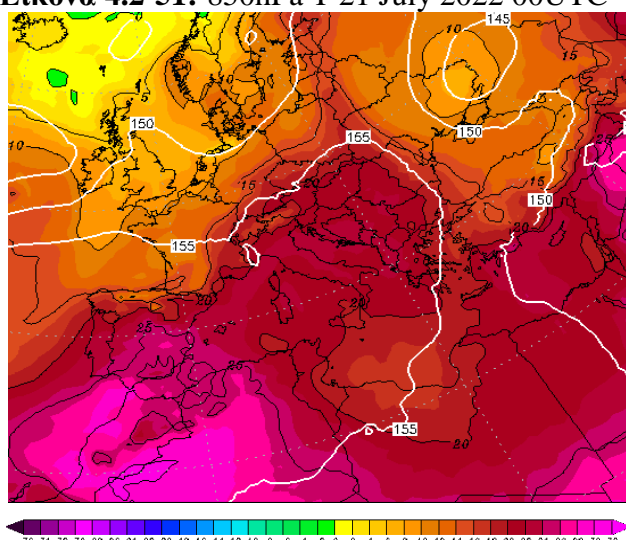
Εικόνα 4.2-53: 850hPa T 23 July 2022 00UTC
