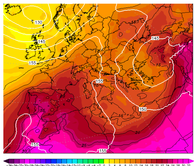
Εικόνα 4.2-12: 850hPa T 12 June 2022 00UTC
