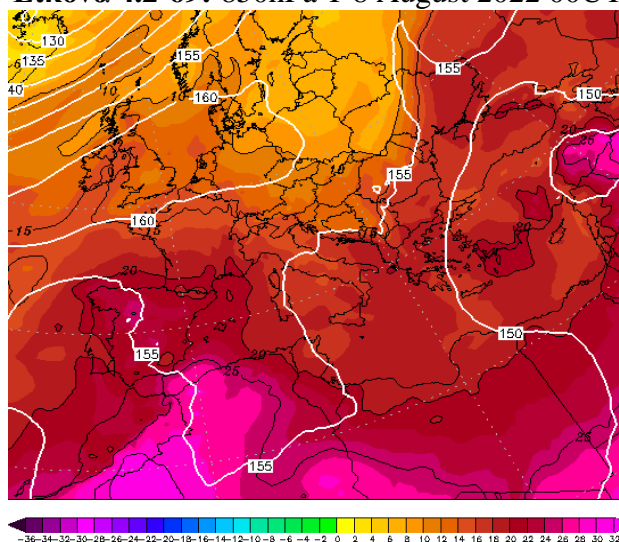
Εικόνα 4.2-71: 850hPa T 10 August 2022 00UTC
