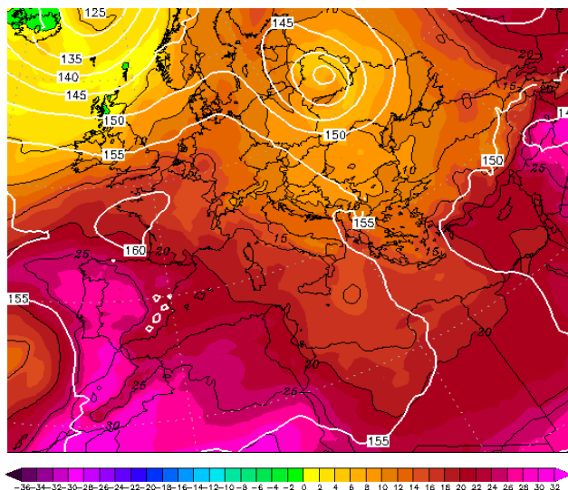
Εικόνα 4.2-43: 850hPa T 13 July 2022 00UTC
