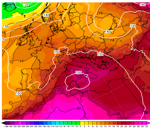
Εικόνα 4.2-23: 850hPa T 23 June 2022 00UTC
