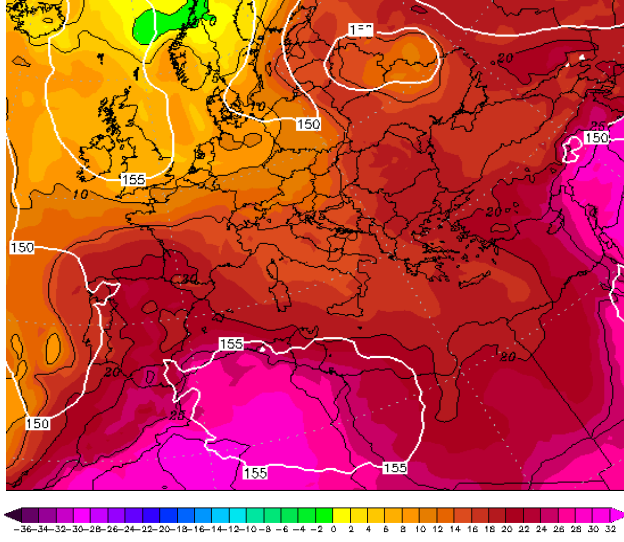
Εικόνα 4.2-90: 850hPa T 29 August 2022 00UTC
