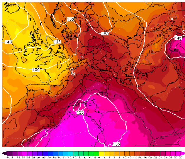
Εικόνα 4.2-31: 850hPa T 1 July 2022 00UTC
