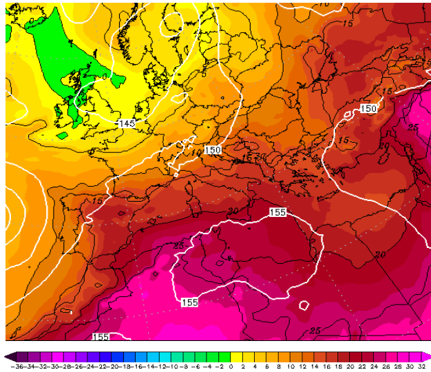
Εικόνα 4.2-1: 850hPa T 1 June 2022 00UTC
