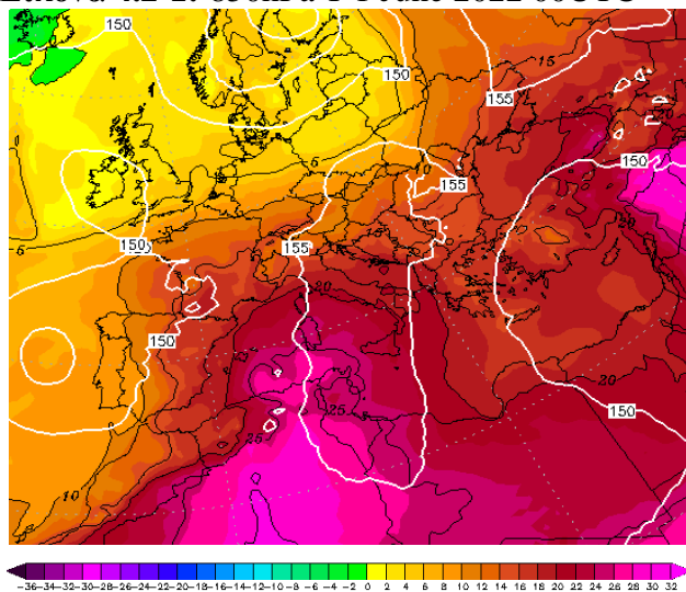
Εικόνα 4.2-3: 850hPa T 3 June 2022 00UTC
