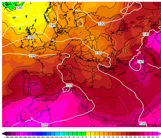
Εικόνα 4.2-62: 850hPa T 1 August 2022 00UTC
