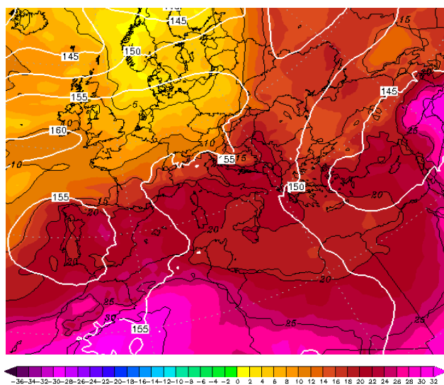
Εικόνα 4.2-68: 850hPa T 7 August 2022 00UTC
