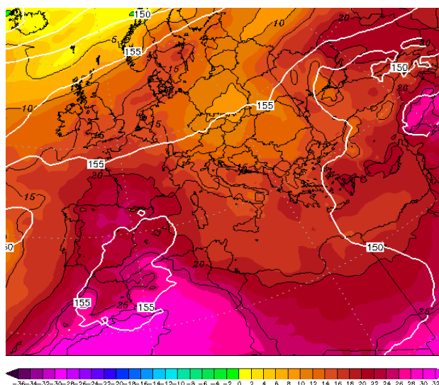
Εικόνα 4.2-73: 850hPa T 12 August 2022 00UTC
