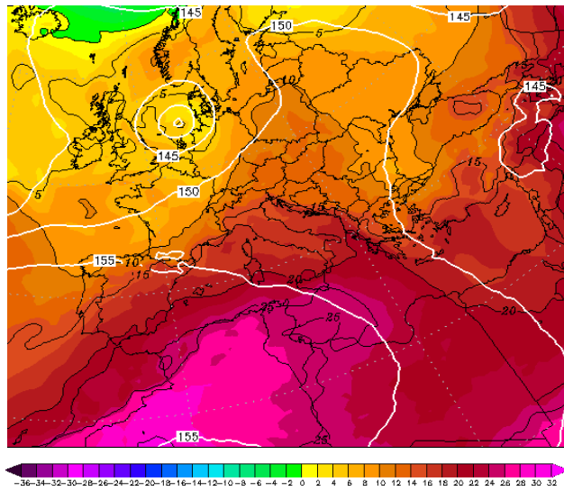
Εικόνα 4.2-7: 850hPa T 7 June 2022 00UTC
