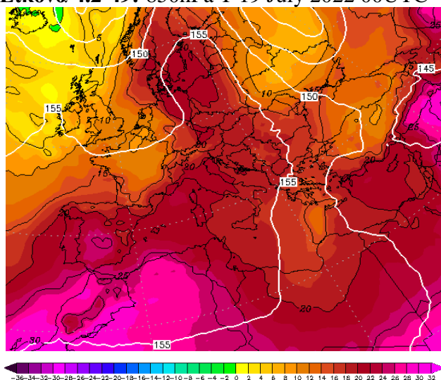
Εικόνα 4.2-51: 850hPa T 21 July 2022 00UTC
