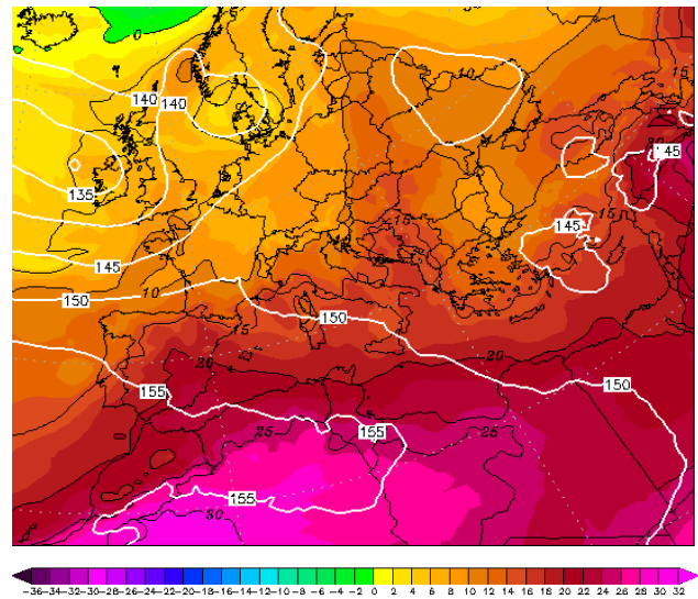
Εικόνα 4.2-8: 850hPa T 8 June 2022 00UTC
