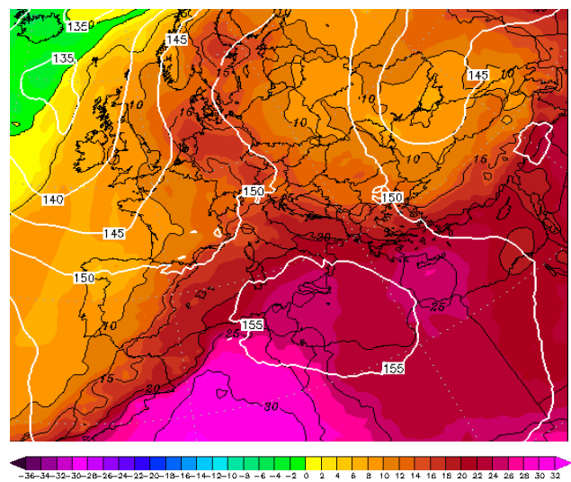
Εικόνα 4.2-24: 850hPa T 24 June 2022 00UTC
