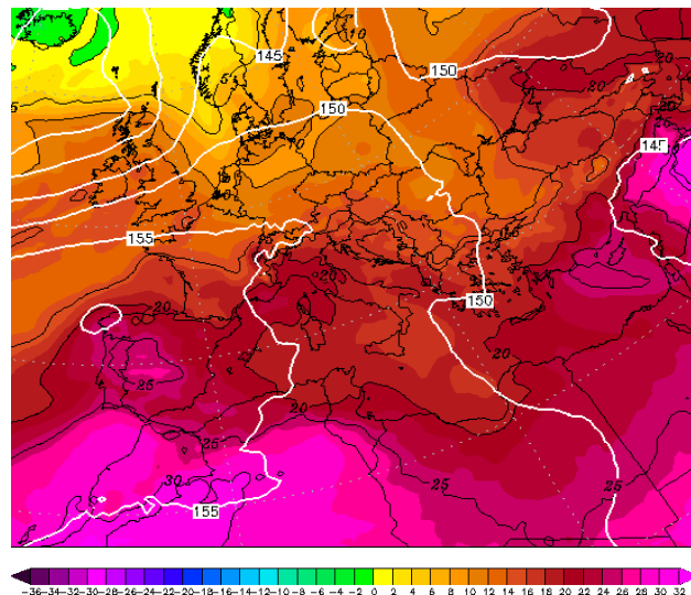
Εικόνα 4.2-63: 850hPa T 2 August 2022 00UTC
