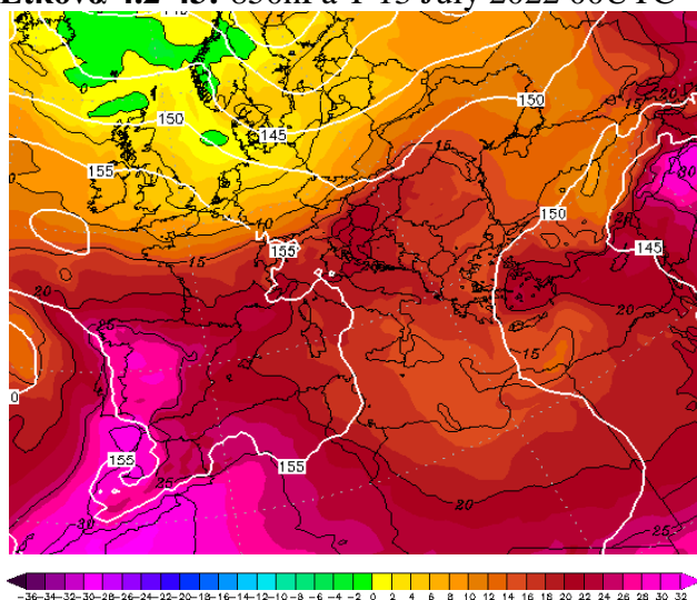
Εικόνα 4.2-45: 850hPa T 15 July 2022 00UTC
