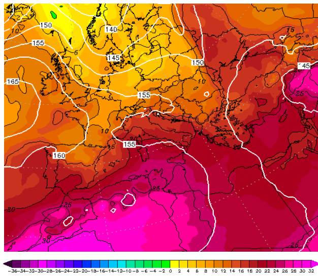
Εικόνα 4.2-37: 850hPa T 7 July 2022 00UTC
