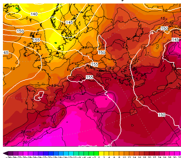
Εικόνα 4.2-36: 850hPa T 6 July 2022 00UTC
