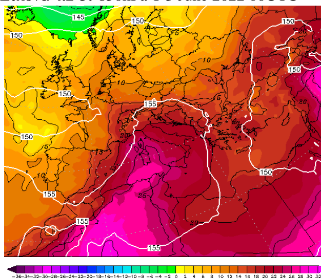
Εικόνα 4.2-5: 850hPa T 5 June 2022 00UTC
