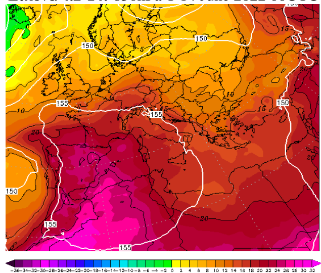
Εικόνα 4.2-16: 850hPa T 16 June 2022 00UTC
