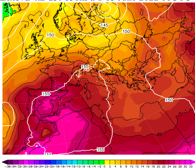
Εικόνα 4.2-15: 850hPa T 15 June 2022 00UTC
