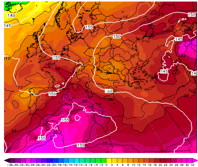
Εικόνα 4.2-75: 850hPa T 14 August 2022 00UTC
