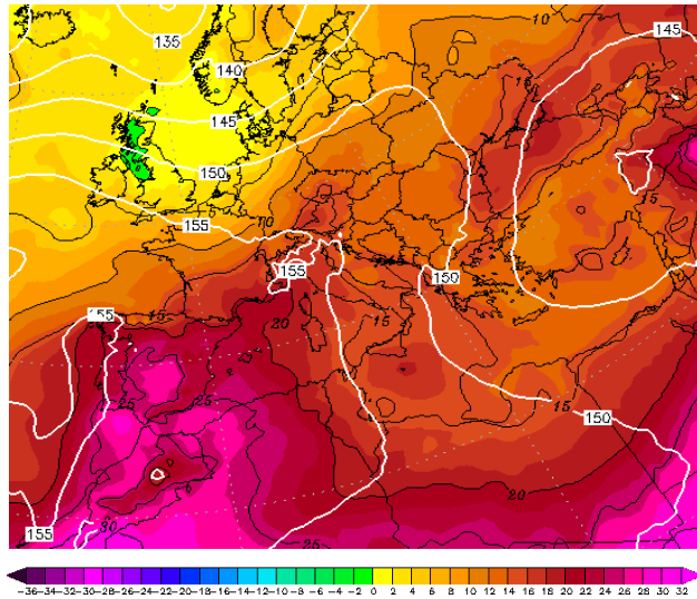
Εικόνα 4.2-13: 850hPa T 13 June 2022 00UTC
