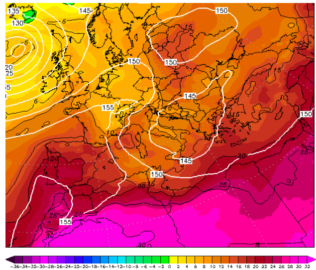
Εικόνα 4.2-10: 850hPa T 10 June 2022 00UTC
