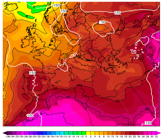
Εικόνα 4.2-89: 850hPa T 28 August 2022 00UTC
