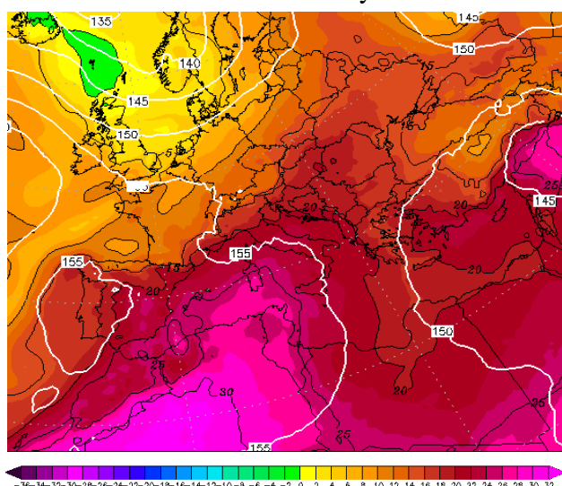
Εικόνα 4.2-35: 850hPa T 5 July 2022 00UTC
