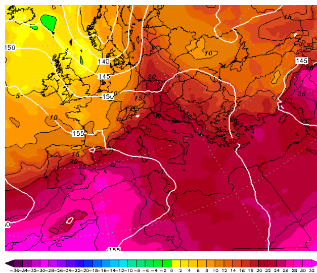
Εικόνα 4.2-56: 850hPa T 26 July 2022 00UTC
