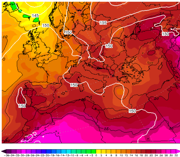
Εικόνα 4.2-88: 850hPa T 27 August 2022 00UTC
