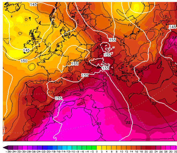
Εικόνα 4.2-32: 850hPa T 2 July 2022 00UTC
