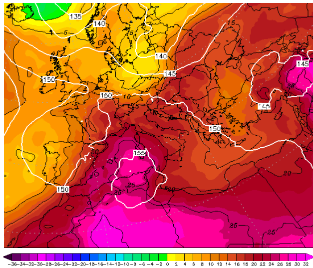
Εικόνα 4.2-21: 850hPa T 21 June 2022 00UTC
