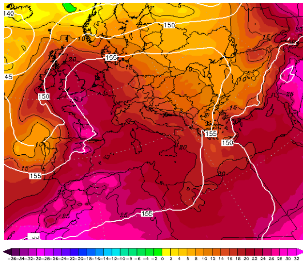
Εικόνα 4.2-49: 850hPa T 19 July 2022 00UTC
