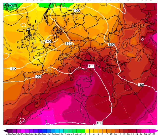
Εικόνα 4.2-6: 850hPa T 6 June 2022 00UTC
