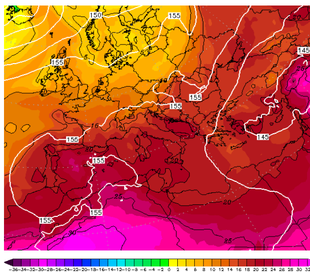
Εικόνα 4.2-69: 850hPa T 8 August 2022 00UTC
