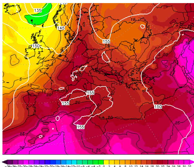
Εικόνα 4.2-66: 850hPa T 5 August 2022 00UTC
