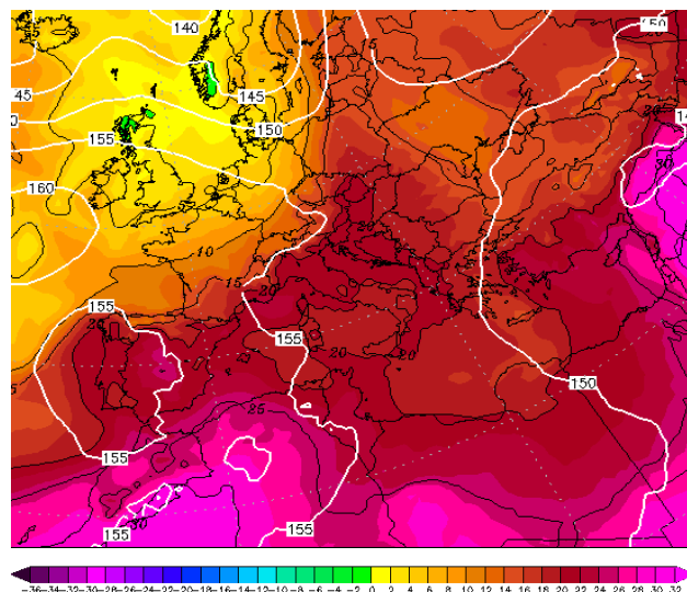
Εικόνα 4.2-67: 850hPa T 6 August 2022 00UTC
