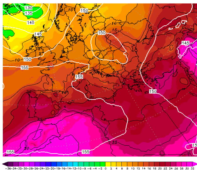
Εικόνα 4.2-61: 850hPa T 31 July 2022 00UTC
