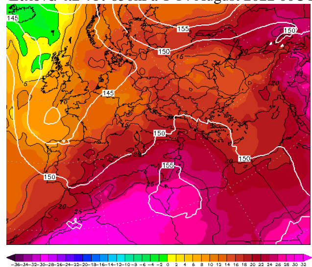
Εικόνα 4.2-77: 850hPa T 16 August 2022 00UTC
