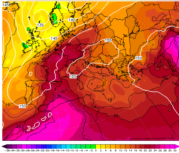
Εικόνα 4.2-19: 850hPa T 19 June 2022 00UTC
