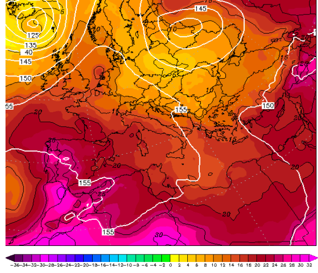
Εικόνα 4.2-42: 850hPa T 12 July 2022 00UTC
