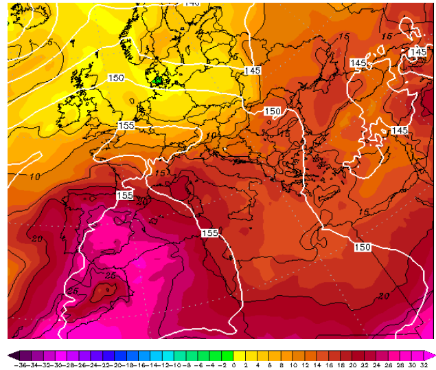
Εικόνα 4.2-14: 850hPa T 14 June 2022 00UTC
