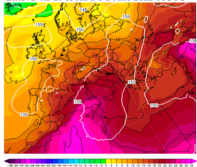
Εικόνα 4.2-4: 850hPa T 4 June 2022 00UTC
