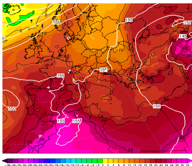
Εικόνα 4.2-72: 850hPa T 11 August 2022 00UTC
