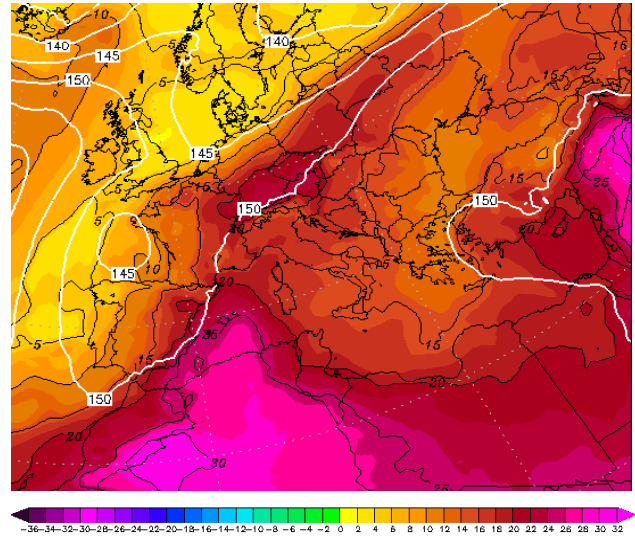
Εικόνα 4.2-20: 850hPa T 20 June 2022 00UTC
