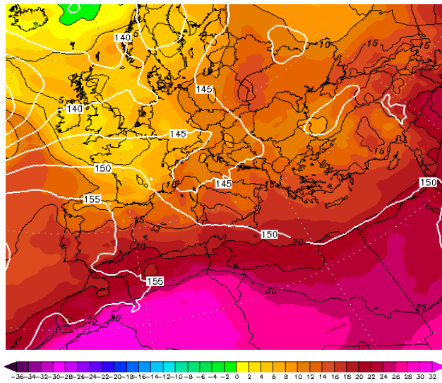
Εικόνα 4.2-9: 850hPa T 9 June 2022 00UTC
