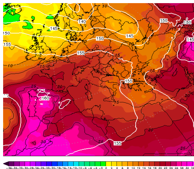
Εικόνα 4.2-44: 850hPa T 14 July 2022 00UTC
