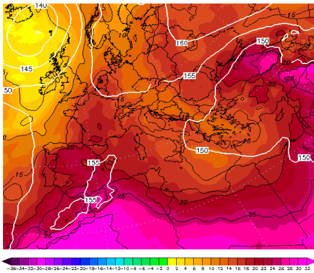
Εικόνα 4.2-86: 850hPa T 25 August 2022 00UTC
