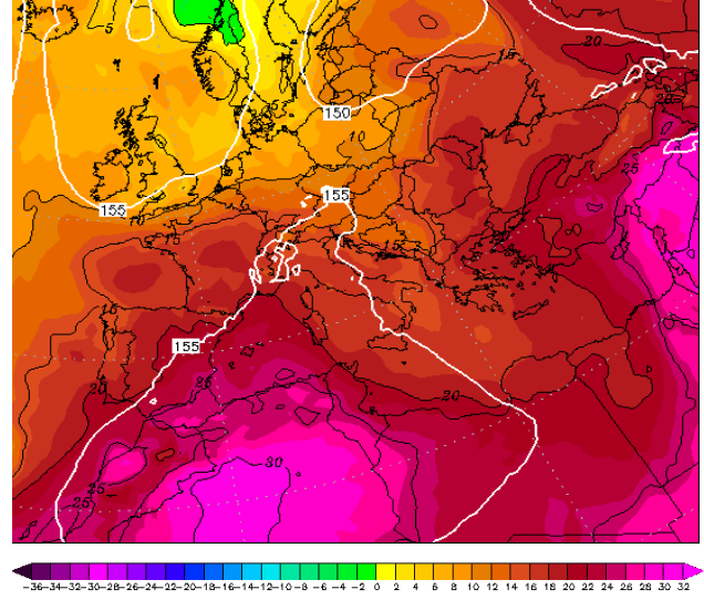
Εικόνα 4.2-91: 850hPa T 30 August 2022 00UTC
