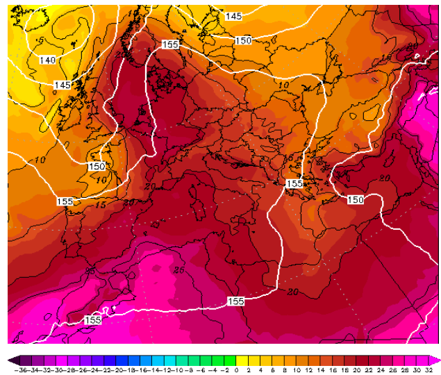
Εικόνα 4.2-50: 850hPa T 20 July 2022 00UTC
