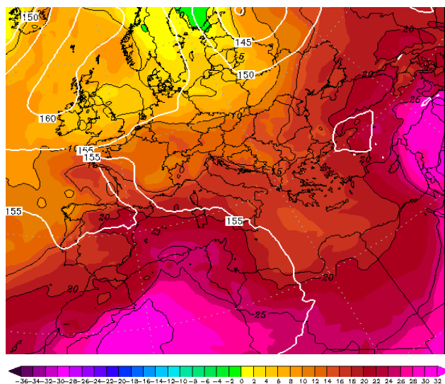
Εικόνα 4.2-92: 850hPa T 31 August 2022 00UTC
