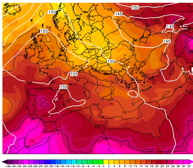
Εικόνα 4.2-41: 850hPa T 11 July 2022 00UTC
