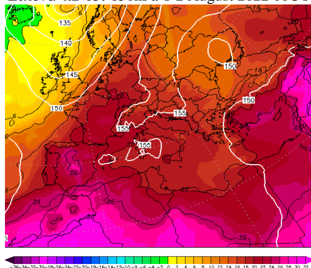
Εικόνα 4.2-65: 850hPa T 4 August 2022 00UTC
