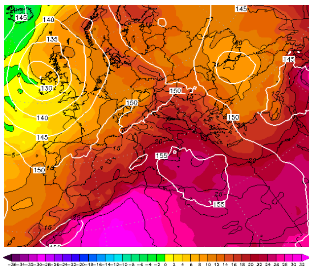
Εικόνα 4.2-25: 850hPa T 25 June 2022 00UTC
