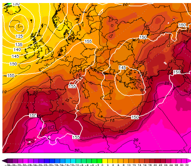
Εικόνα 4.2-11: 850hPa T 11 June 2022 00UTC
