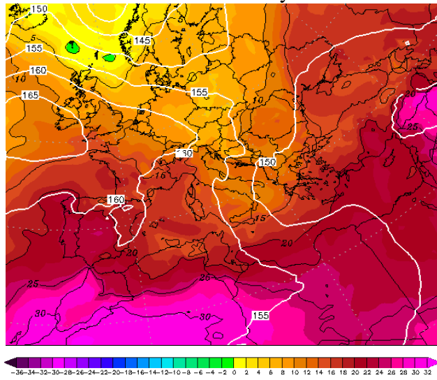
Εικόνα 4.2-39: 850hPa T 9 July 2022 00UTC
